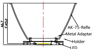
光学装配示意图
